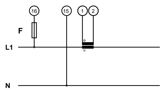
Monofase, 2 fili, connessione con 1 TA
