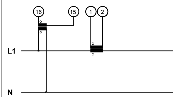
Monofase, 2 fili, connessione con 1 TA e 1 TV
